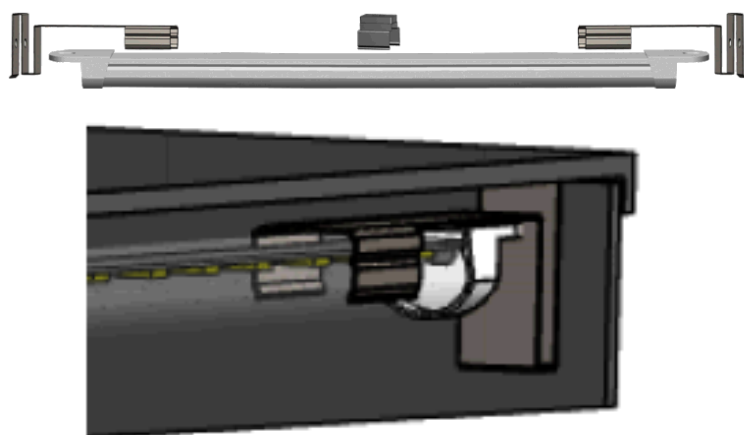
Рис. 22 - Вид для замены светильника в общем верхнем плафоне
