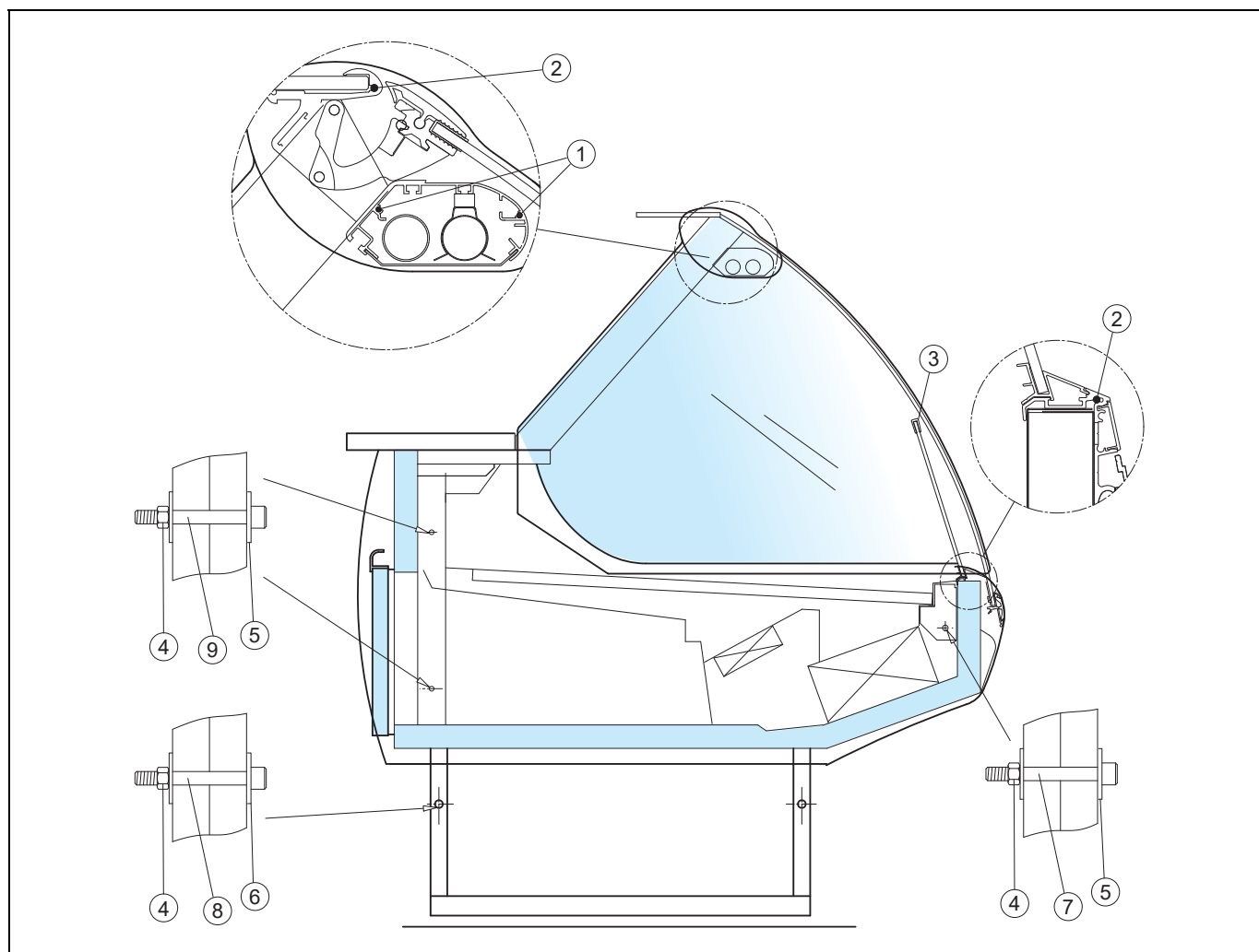
Рис. 11 Схема соединения витрин в канал.
