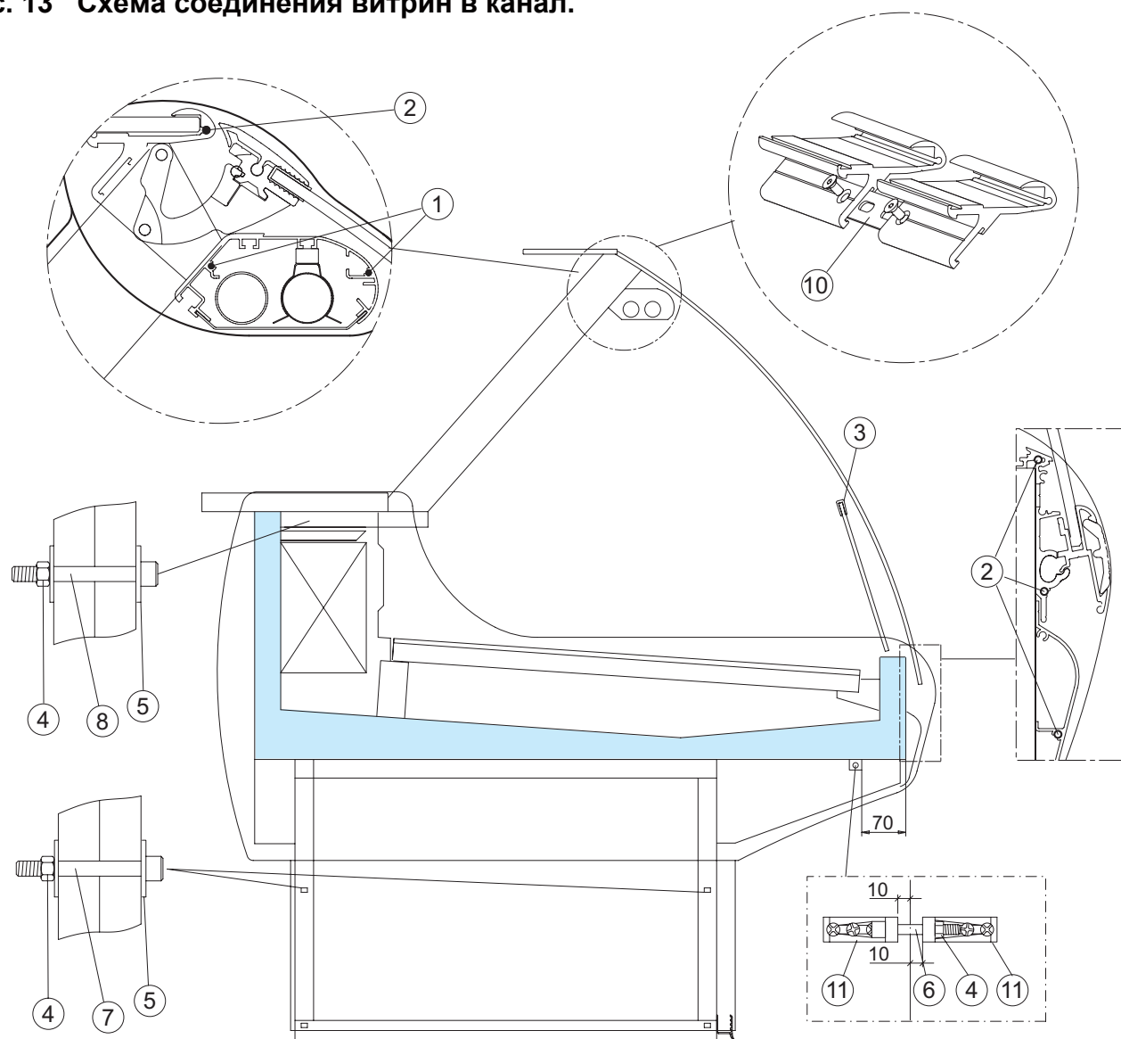
Рис. 13 Схема соединения витрин в канал.
