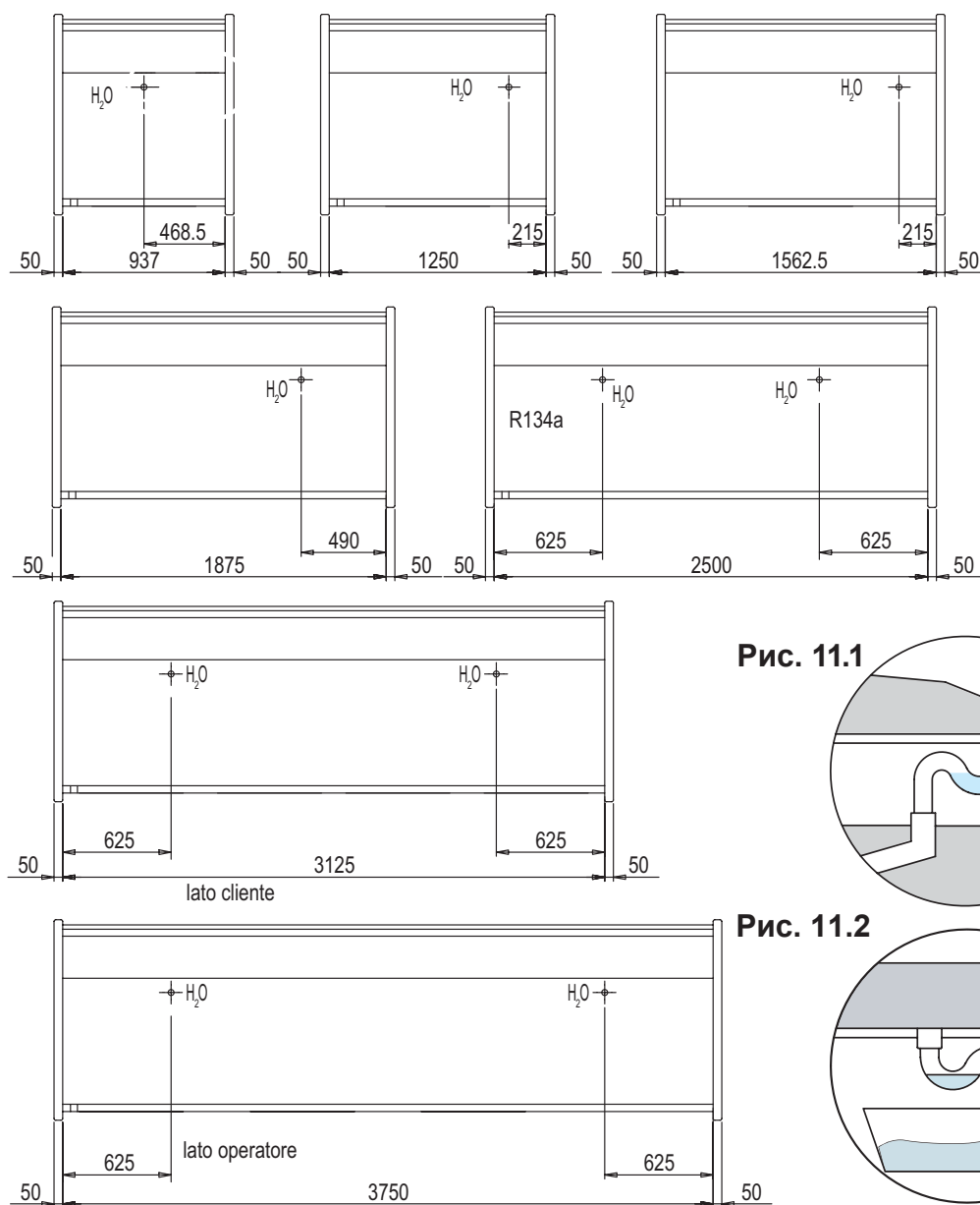
Рис.11 Оттайка и дренаж
